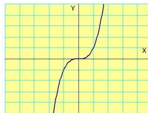
Función f(x)=x^3
