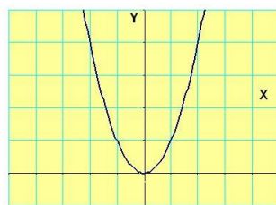
Función f(x)=x^2
