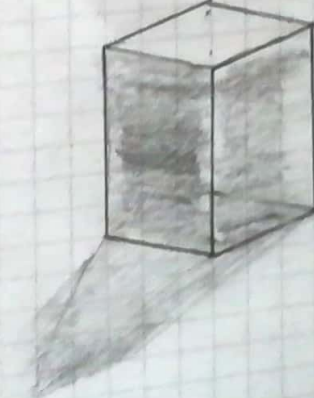
Paralelogramo
