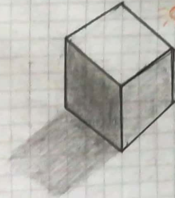
cubo
