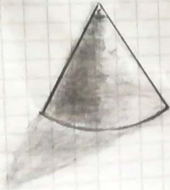
cono
