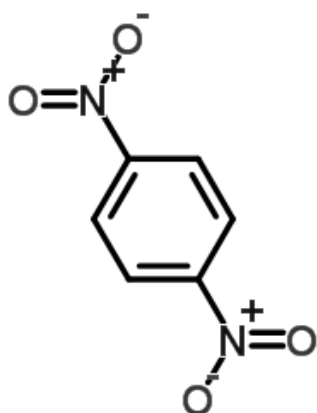
p-.dinitrobenceno
