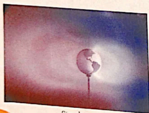
Simulación de los Cinturón Van Allen, imagen tomada de la NASA.
